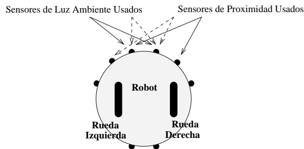
Figura 4: Distribución de los sensores usados en el experimento.
