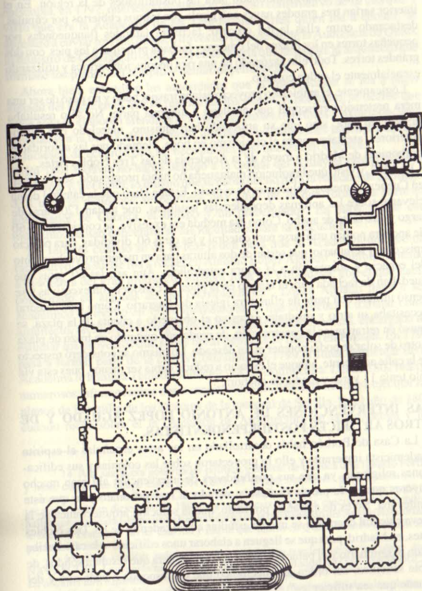
Plano 2. Plano de la catedral de Málaga.
