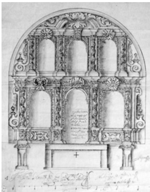
Fig. 4. ¿Domingo de Andrade?, trazas para el retablo mayor de San Lourenzo de Trasouto (Santiago de Compostela), ¿1700 ca.?, [vid. A. VIGO TRASANCOS (dir.), Planos y dibujos de arquitectura y urbanismo: Galicia en los siglos XVI y XVII , Santiago de Compostela, Consello Galego de Colexios de Aparelladores e Arquitectos Técnicos, 2003, Dib/185, ilustr. 513 p.]
