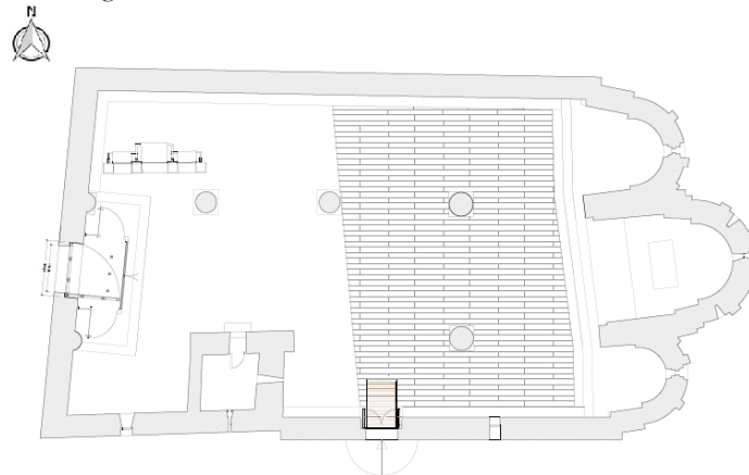
Figura 6.5: Planta de Santa María de Tahüll
