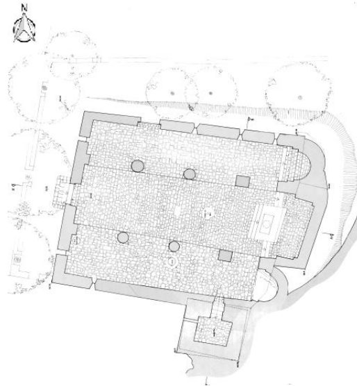
Figura 6.6: Planta de Sant Joan de Bohí
